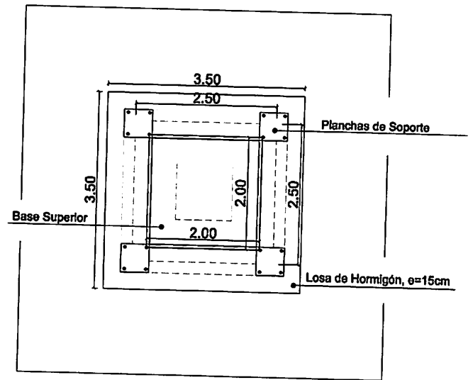
Vista en Planta, Esc 1:100
